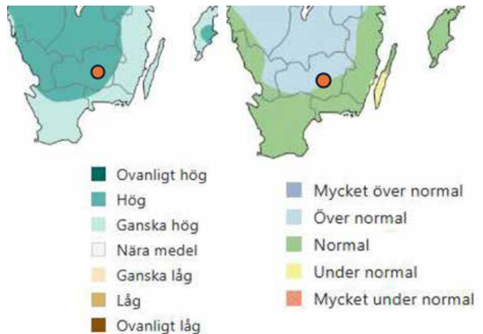
Figur 2: Bild visar grundvattennivå vecka 6 i jämförelse med samtliga nivåer för perioden 1961-2024 (SGU)
