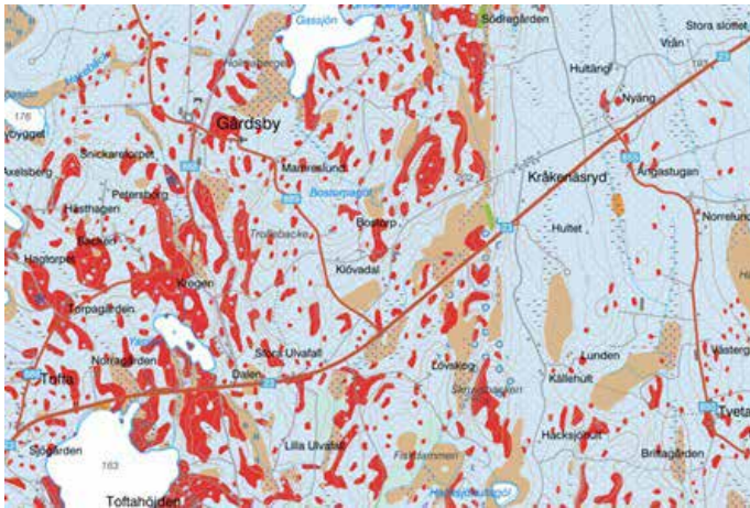
Figur 1: Utdrag ur SGU jordartskarta (2025).
